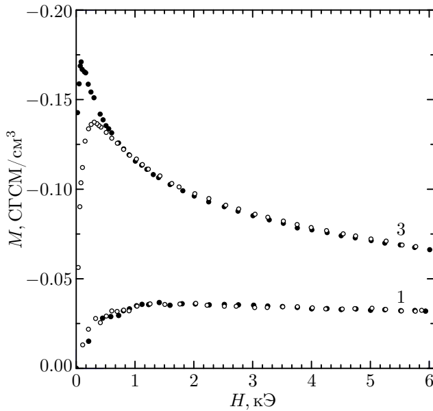
Рис. 3. Зависимости намагниченности образцов 1 и 3 от магнитного поля при температуре 90 К. Закрытые символы — увеличение магнитного поля, открытые — его уменьшение. Цифры — номера образцов
