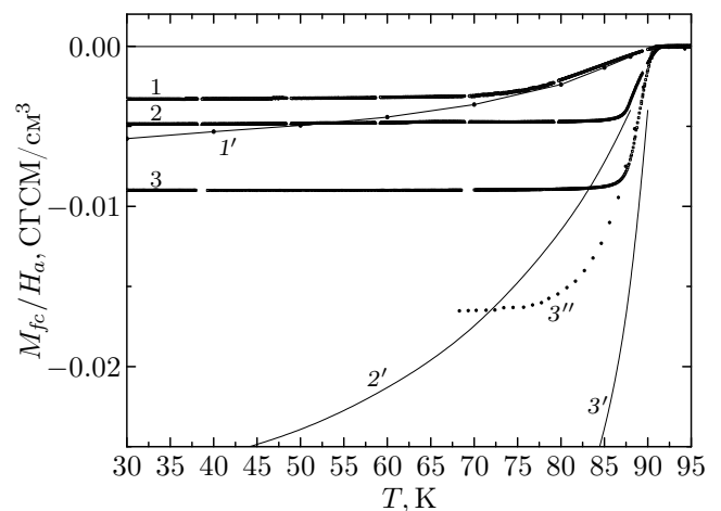
Рис. 2. Зависимость намагниченности M_{fc} от температуры при охлаждении в постоянном магнитном поле H_a = 10 Э образцов 1, 2, 3 (расчет с учетом рентгеновской плотности). Цифры — номера образцов. Кривая 1' — расчет по квазилинейному участку M(H) для образца 1, Кривые 2' и 3' — расчет по данным [11], 3'' — экспериментальная зависимость M_{fc} в поле H_a = 53.3 Э
