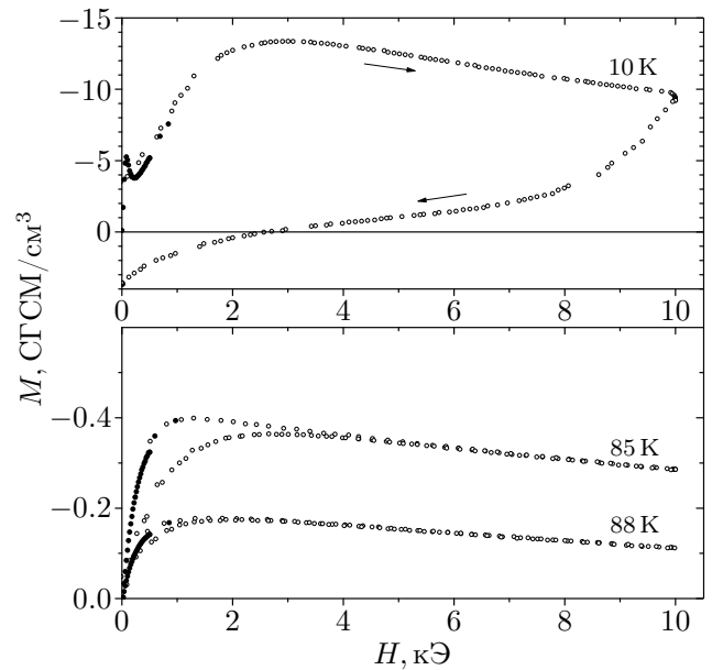
Рис. 4. Зависимость намагниченности образца 1 от магнитного поля при температурах 10, 85 и 88 К. Закрытыми символами приведены начальные участки кривой первого ввода поля
