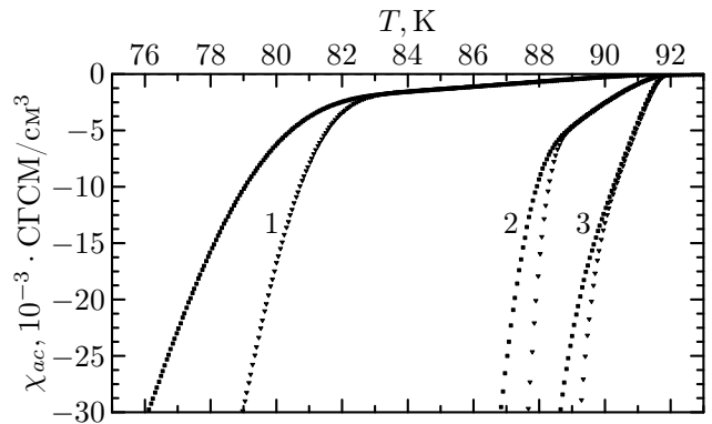
Рис. 6. Зависимости \chi_{ac} от температуры в переменных магнитных полях образцов 1, 2, 3 по данным [12]
